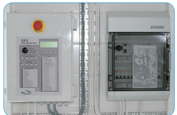
Förbränningsautomatik SA2.
